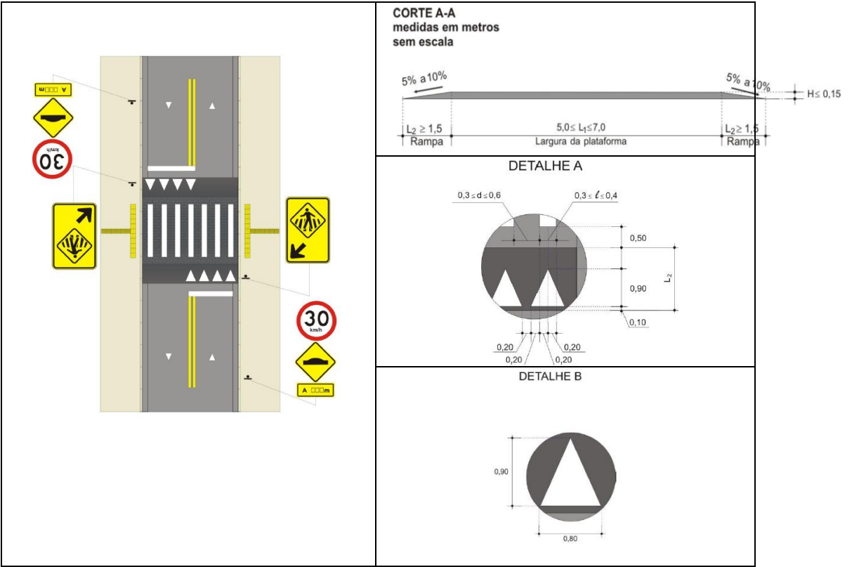
Figura 1 - Conjunto do dispositivo com faixa elevada
