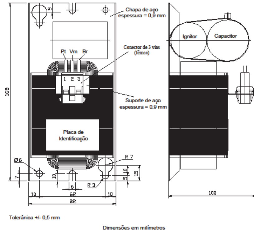
Figura 2: Kit removível para luminárias integradas para lâmpadas VS 250 W.
