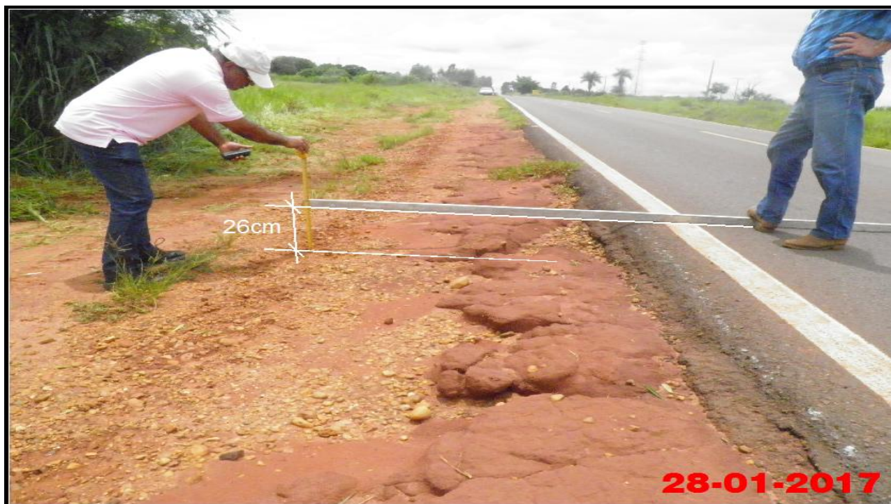
Foto 17 – Vista geral do desnível da Rodovia Arlindo Bértio (SP-613) com o seu acostamento do lado esquerdo no sentido à Rosana.
