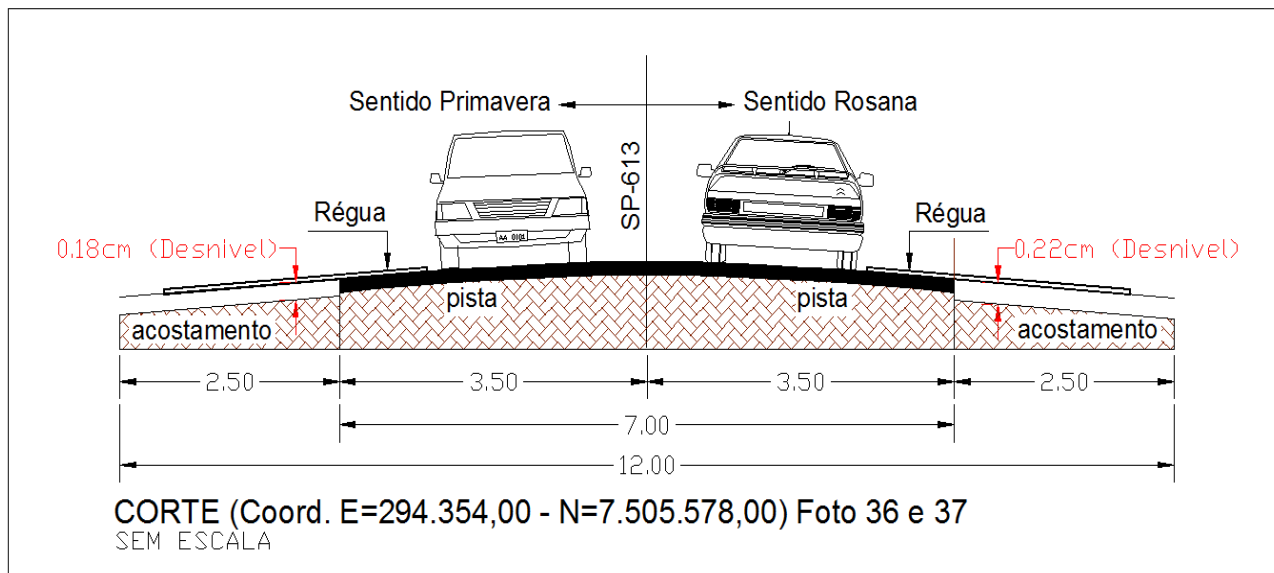
Figura 23 – Desenho do Corte da Rodovia Arlindo Bértio (SP-613), demonstrando o desnível da Rodovia com o seu acostamento do lado direito e esquerdo no sentido Euclides da Cunha Paulista à Rosana.
