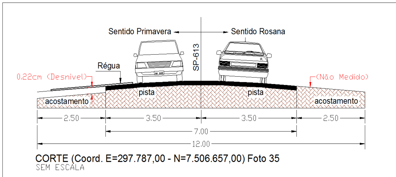
Figura 22 – Desenho do Corte da Rodovia Arlindo Bértio (SP-613), demonstrando o desnível da Rodovia com o seu acostamento do lado esquerdo no sentido Euclides da Cunha Paulista à Rosana.
