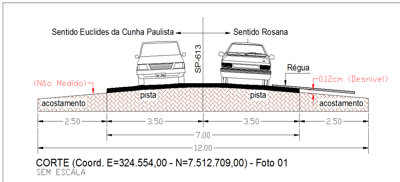
Figura 02 – Desenho do Corte da Rodovia Arlindo Bétio (SP-613), demonstrando o desnível da Rodovia com o seu acostamento do lado direito no sentido Euclides da Cunha Paulista à Rosana.
