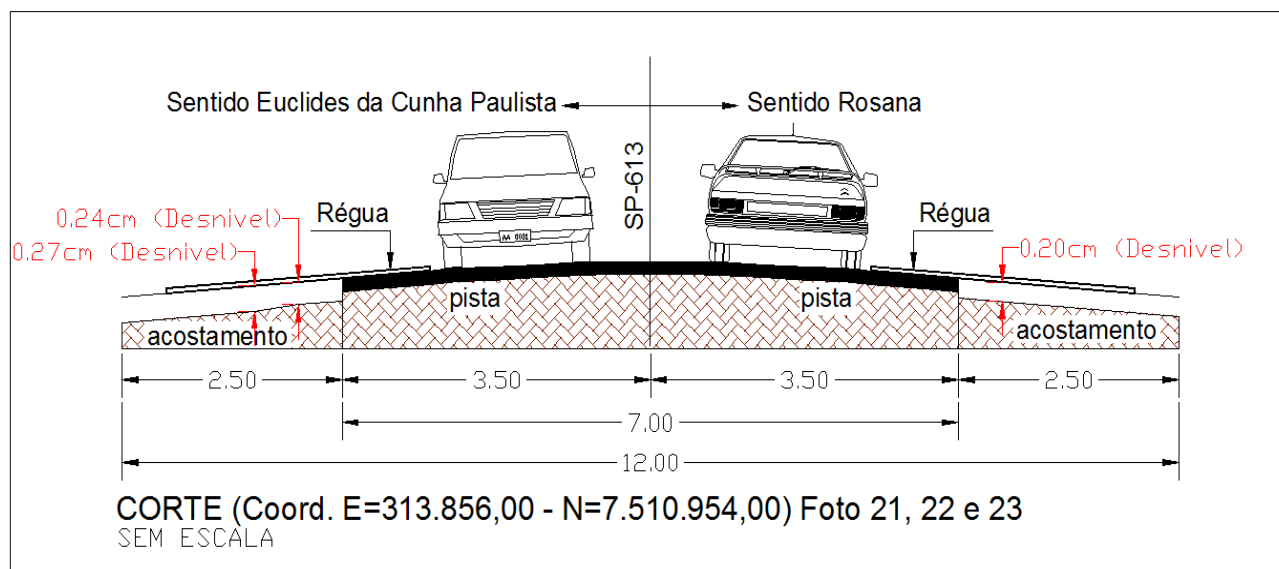
Figura 13 – Desenho do Corte da Rodovia Arlindo Bétio (SP-613), demonstrando o desnível da Rodovia com o seu acostamento do lado direito e esquerdo no sentido Euclides da Cunha Paulista à Rosana.
