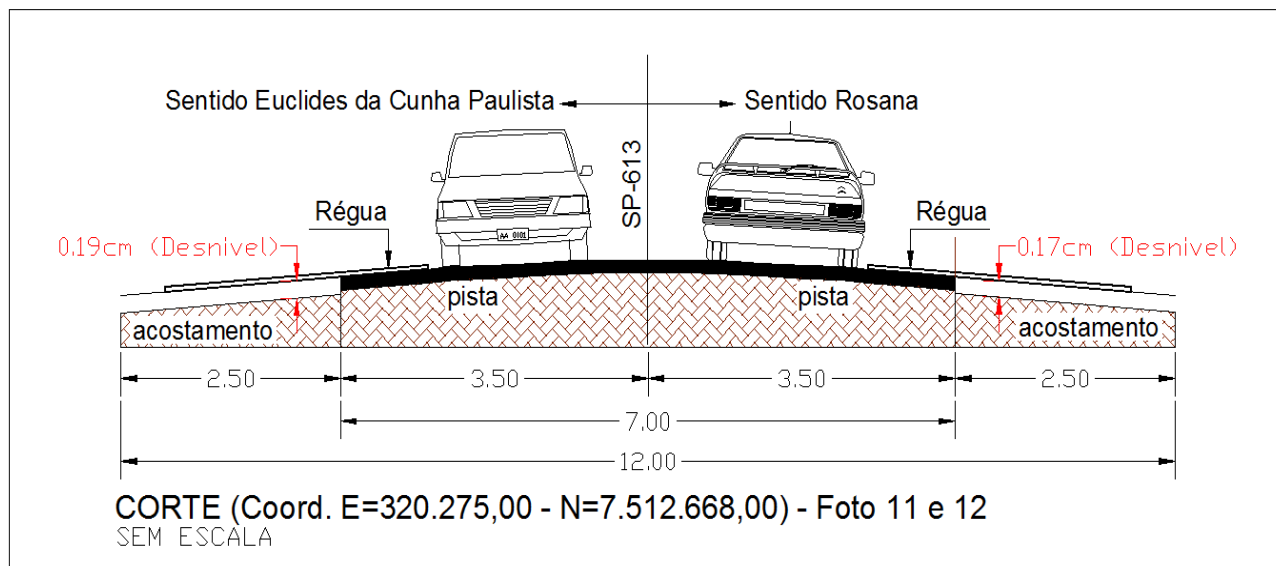
Figura 08 – Desenho do Corte da Rodovia Arlindo Bértio (SP-613), demonstrando o desnível da Rodovia com o seu acostamento do lado direito e esquerdo no sentido Euclides da Cunha Paulista à Rosana.
