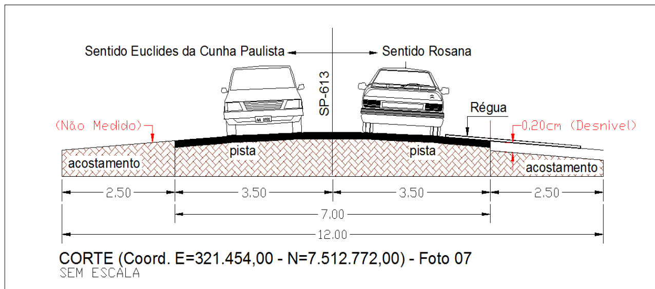
Figura 06 – Desenho do Corte da Rodovia Arlindo Bértio (SP-613), demonstrando o desnível da Rodovia com o seu acostamento do lado direito no sentido Euclides da Cunha Paulista à Rosana.
