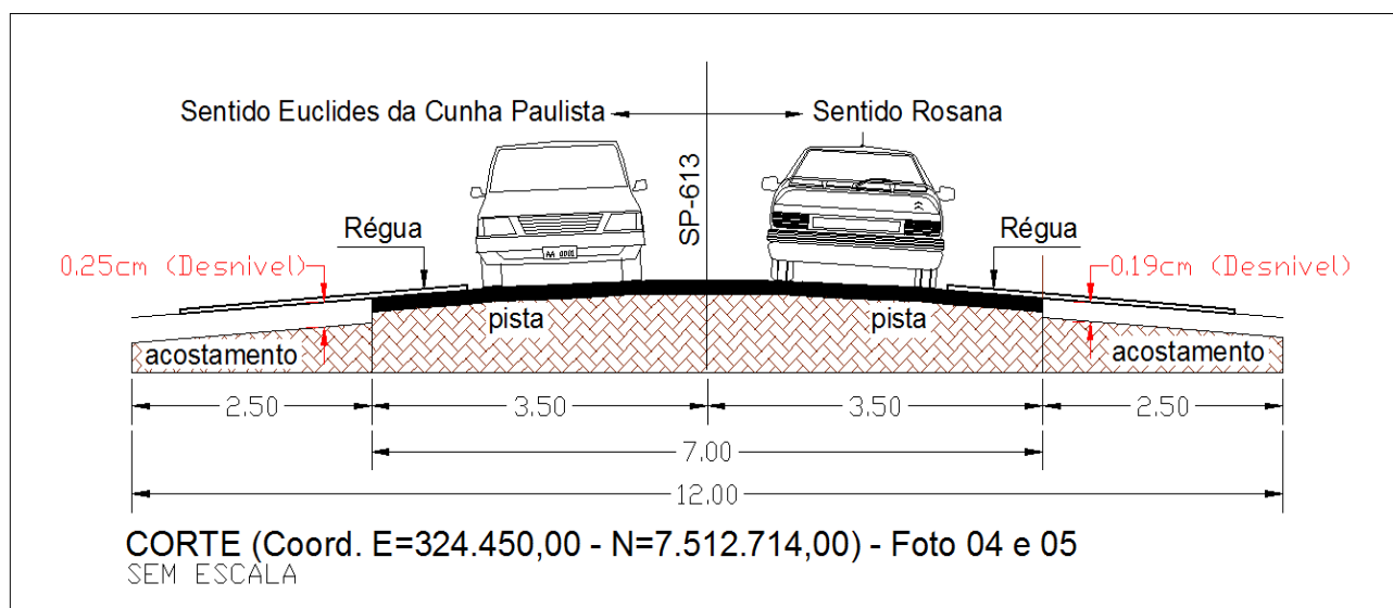
Figura 04 – Desenho do Corte da Rodovia Arlindo Bértio (SP-613), demonstrando o desnível da Rodovia com o seu acostamento do lado direito e esquerdo no sentido Euclides da Cunha Paulista à Rosana.
