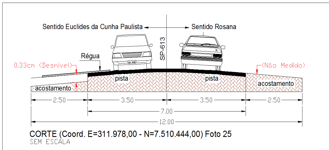
Figura 15 – Desenho do Corte da Rodovia Arlindo Bétio (SP-613), demonstrando o desnível da Rodovia com o seu acostamento do lado esquerdo no sentido Euclides da Cunha Paulista à Rosana.
