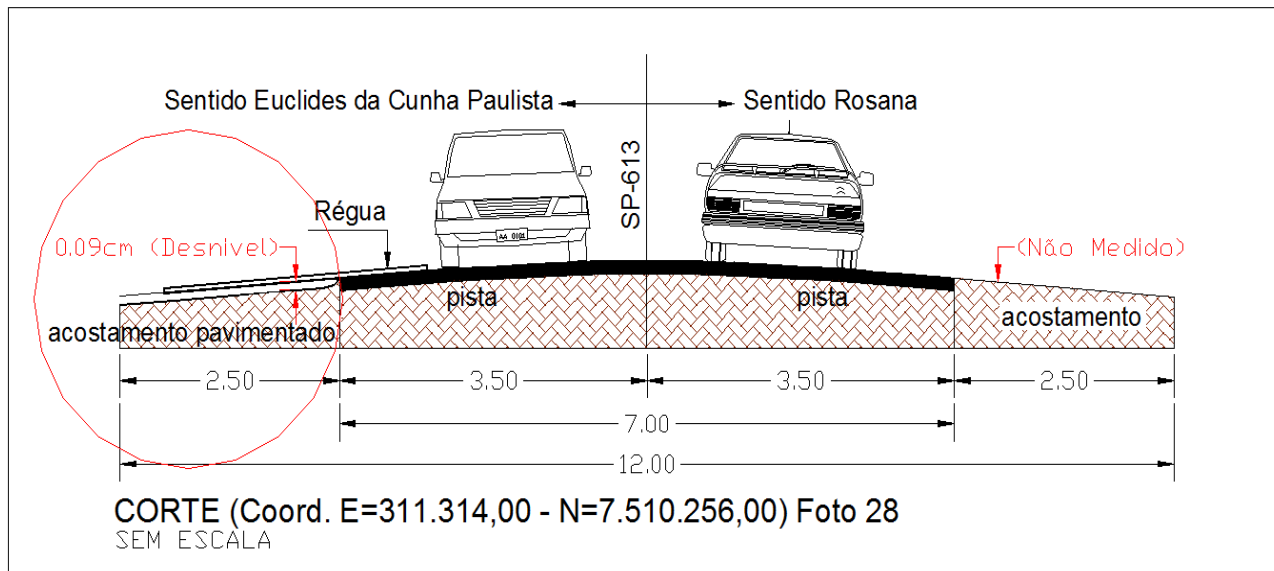
Figura 17 – Desenho do Corte da Rodovia Arlindo Bértio (SP-613), demonstrando o desnível da Rodovia com o seu acostamento do lado esquerdo no sentido Euclides da Cunha Paulista à Rosana.
