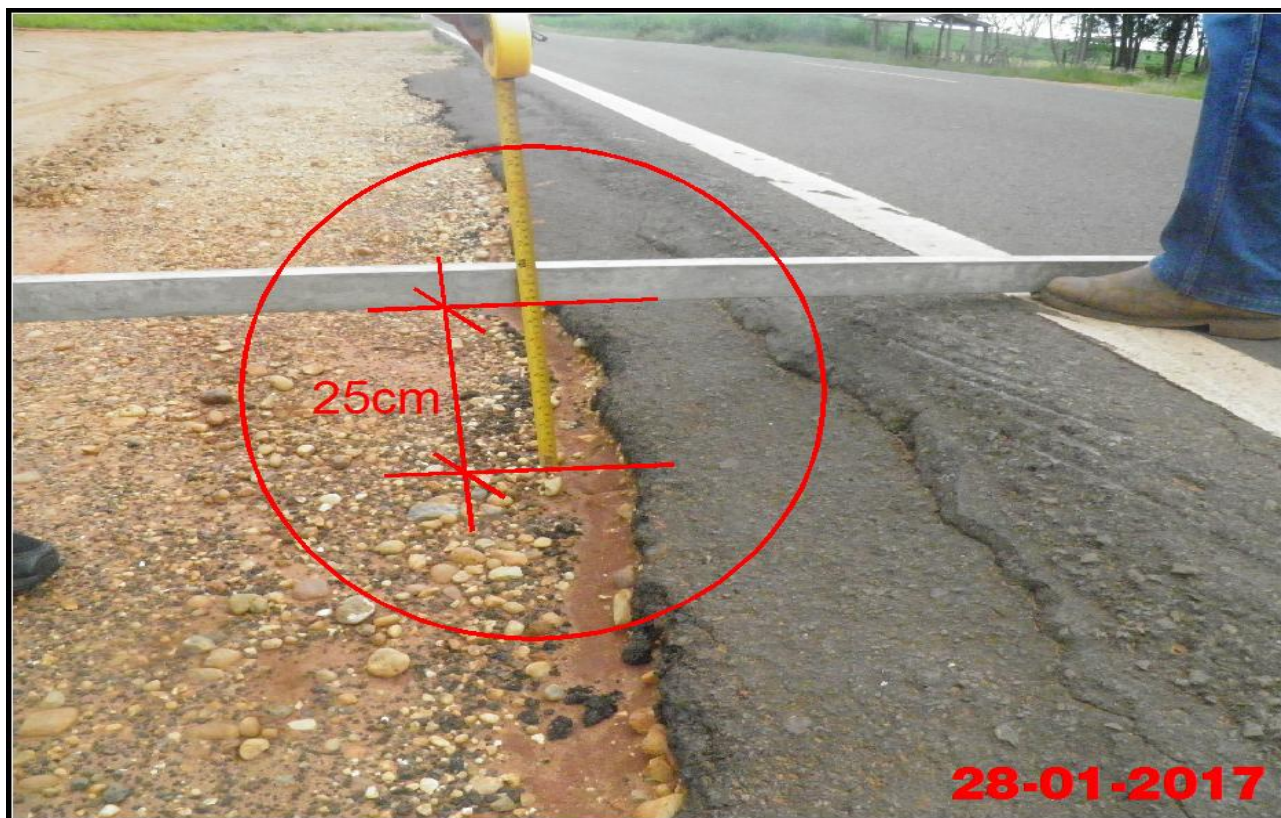
Foto 43 – Vista do Detalhe mostrando o desnível da Rodovia Arlindo Bétio (SP-613) com o seu acostamento do lado direito próximo ao perímetro urbano no sentido à Rosana.
