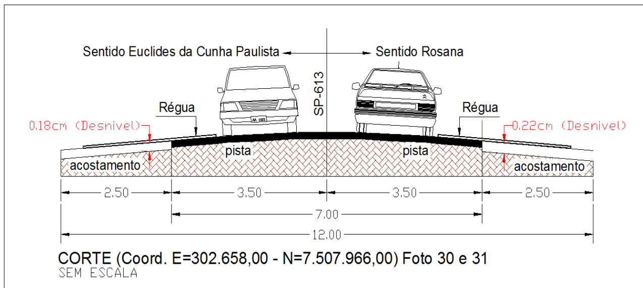
Figura 19 – Desenho do Corte da Rodovia Arlindo Bértio (SP-613), demonstrando o desnível da Rodovia com o seu acostamento do lado direito e esquerdo no sentido Euclides da Cunha Paulista à Rosana.
