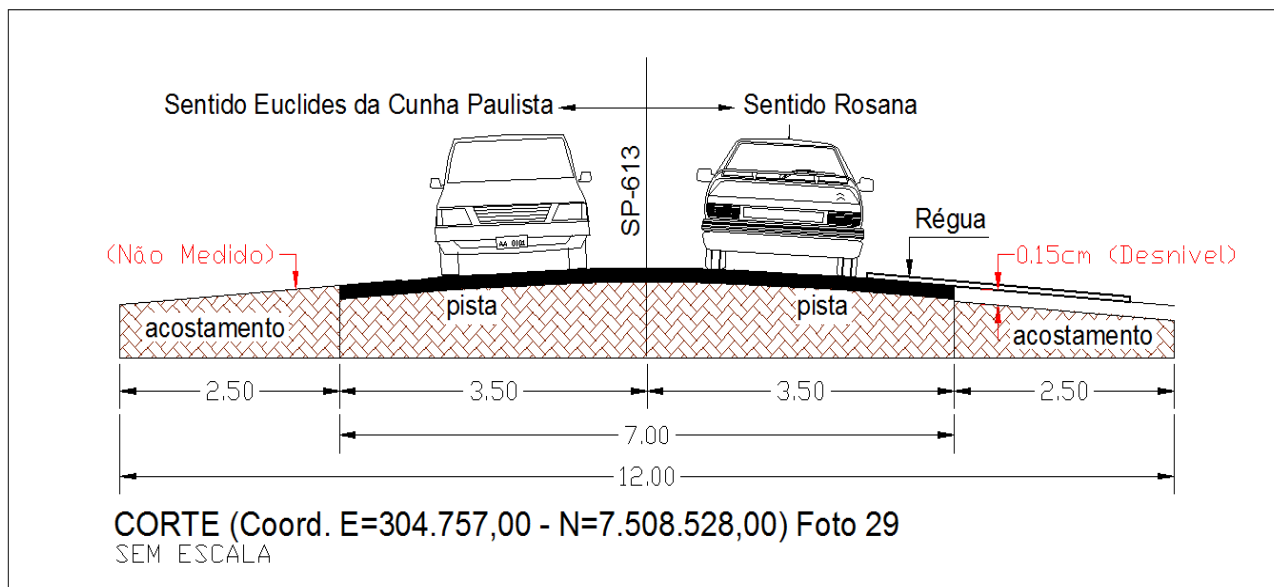
Figura 18 – Desenho do Corte da Rodovia Arlindo Bétio (SP-613), demonstrando o desnível da Rodovia com o seu acostamento do lado direito no sentido Euclides da Cunha Paulista à Rosana.
