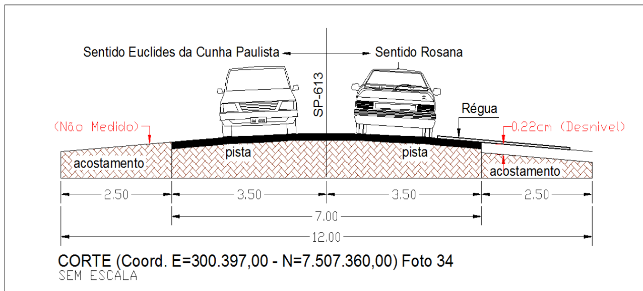
Figura 21 – Desenho do Corte da Rodovia Arlindo Bétio (SP-613), demonstrando o desnível da Rodovia com o seu acostamento do lado direito no sentido Euclides da Cunha Paulista à Rosana.
