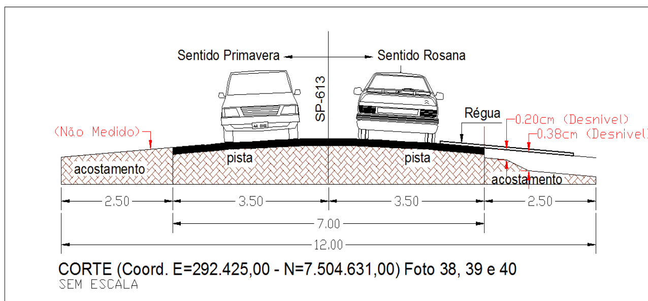
Figura 24 – Desenho do Corte da Rodovia Arlindo Bétio (SP-613), demonstrando o desnível da Rodovia com o seu acostamento do lado direito no sentido Euclides da Cunha Paulista à Rosana.
