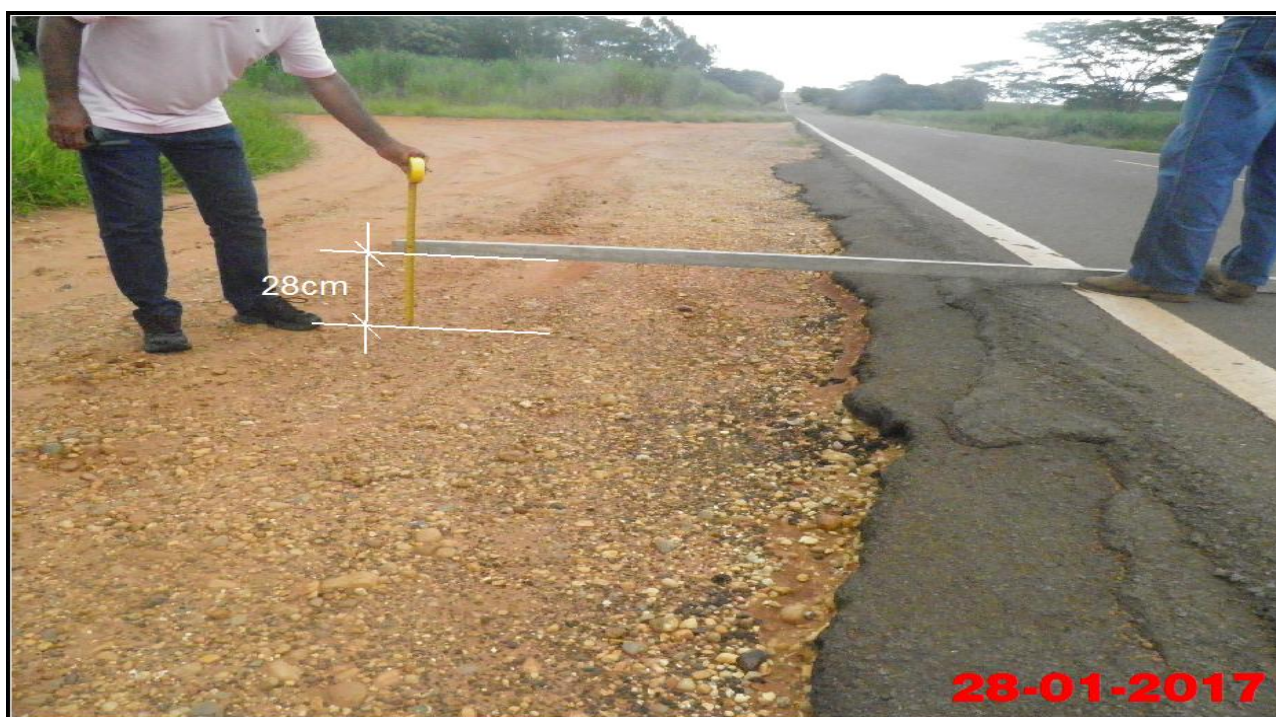
Foto 42 – Vista geral do desnível da Rodovia Arlindo Bértio (SP-613) com o seu acostamento do lado direito no sentido à Rosana.
