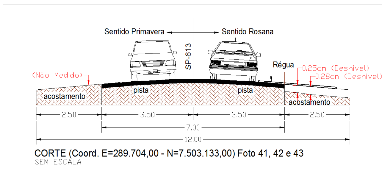
Figura 25 – Desenho do Corte da Rodovia Arlindo Bétio (SP-613), demonstrando o desnível da Rodovia com o seu acostamento do lado direito no sentido Euclides da Cunha Paulista à Rosana.
