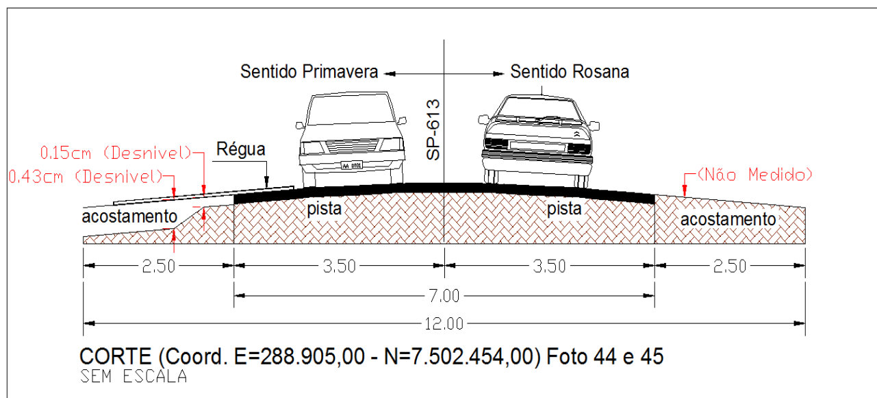
Figura 26 – Desenho do Corte da Rodovia Arlindo Bétio (SP-613), demonstrando o desnível da Rodovia com o seu acostamento do lado esquerdo no sentido Euclides da Cunha Paulista à Rosana.
