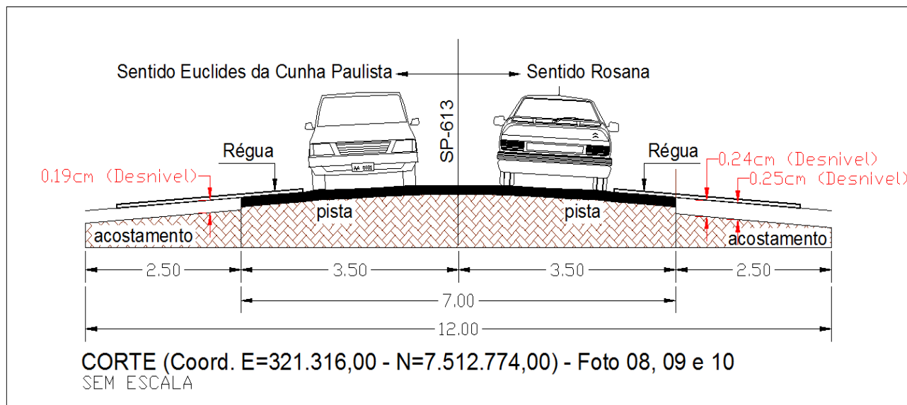
Figura 07 – Desenho do Corte da Rodovia Arlindo Bértio (SP-613), demonstrando o desnível da Rodovia com o seu acostamento do lado direito e esquerdo no sentido Euclides da Cunha Paulista à Rosana.
