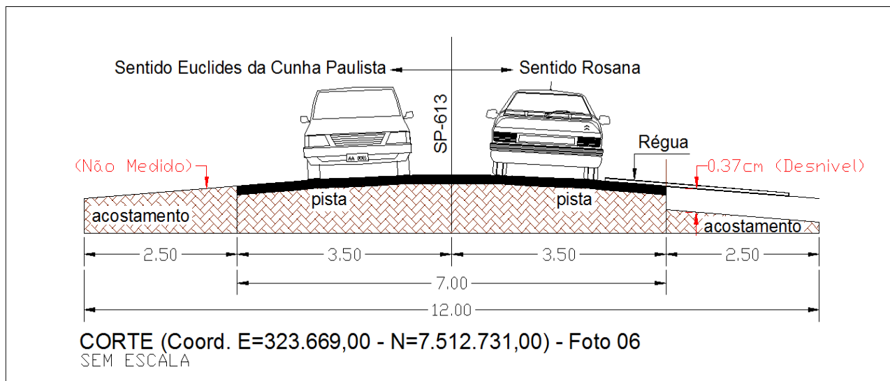
Figura 05 – Desenho do Corte da Rodovia Arlindo Bétio (SP-613), demonstrando o desnível da Rodovia com o seu acostamento do lado direito no sentido Euclides da Cunha Paulista à Rosana.
