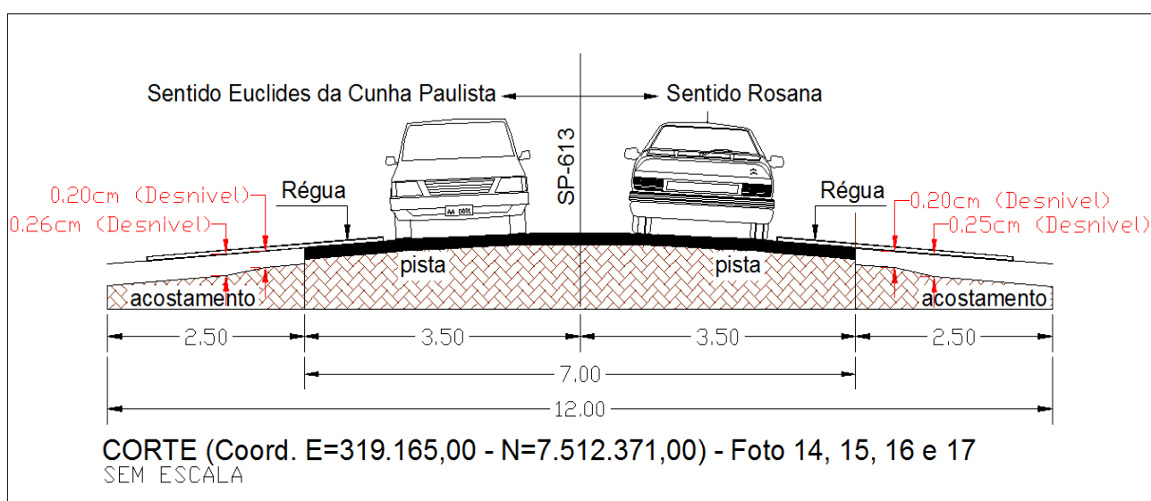
Figura 10 – Desenho do Corte da Rodovia Arlindo Bétio (SP-613), demonstrando o desnível da Rodovia com o seu acostamento do lado direito e esquerdo no sentido Euclides da Cunha Paulista à Rosana.
