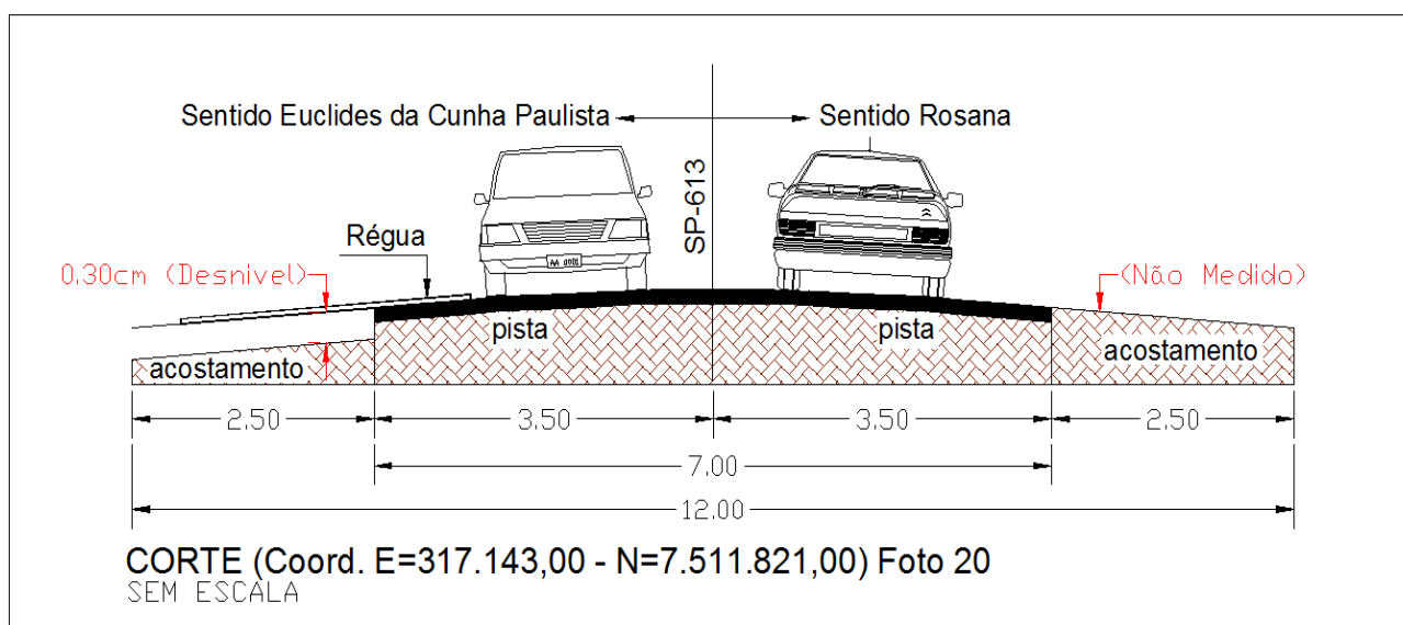
Figura 12 – Desenho do Corte da Rodovia Arlindo Bétio (SP-613), demonstrando o desnível da Rodovia com o seu acostamento do lado esquerdo no sentido Euclides da Cunha Paulista à Rosana.
