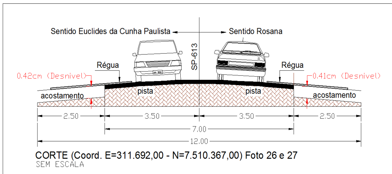
Figura 16 – Desenho do Corte da Rodovia Arlindo Bértio (SP-613), demonstrando o desnível da Rodovia com o seu acostamento do lado direito e esquerdo no sentido Euclides da Cunha Paulista à Rosana.
