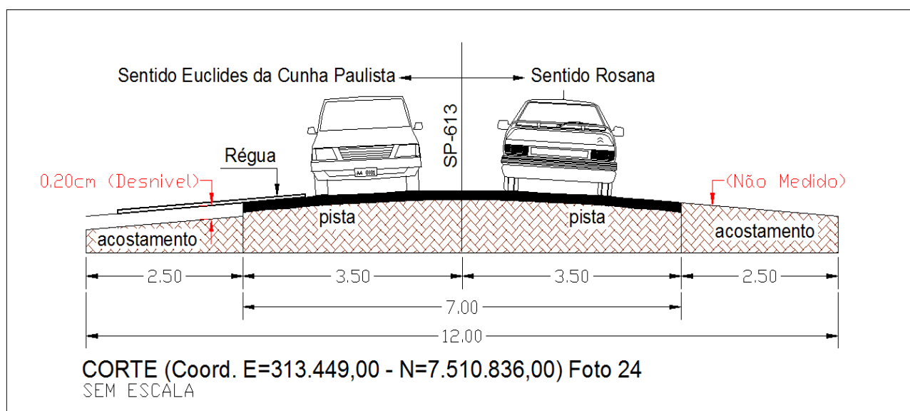
Figura 14 – Desenho do Corte da Rodovia Arlindo Bétio (SP-613), demonstrando o desnível da Rodovia com o seu acostamento do lado esquerdo no sentido Euclides da Cunha Paulista à Rosana.
