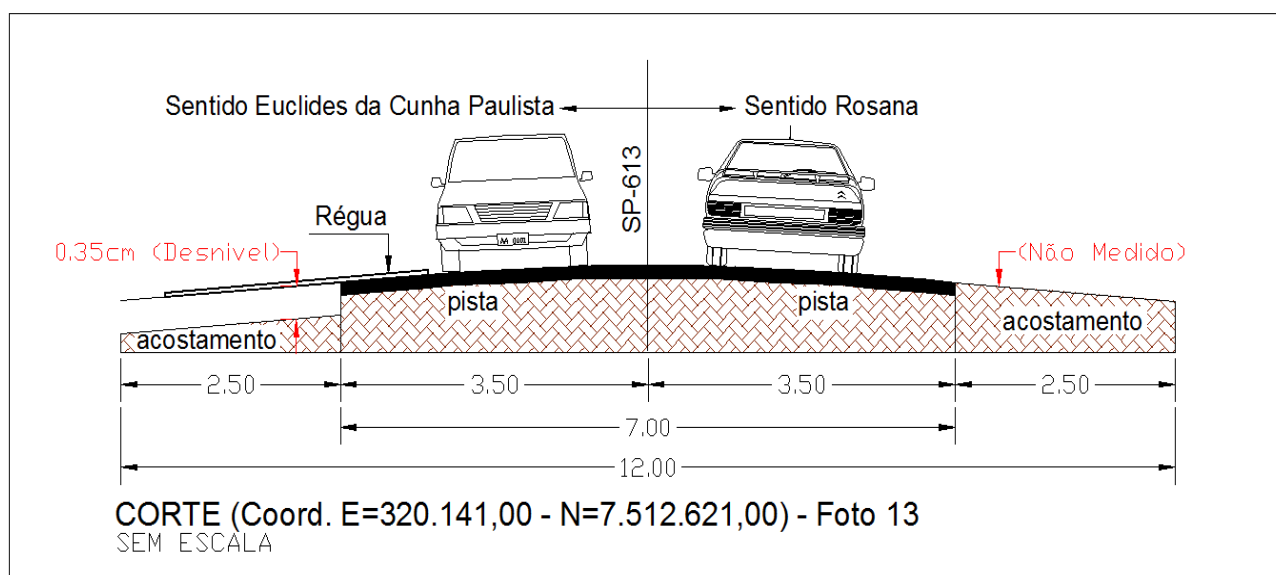
Figura 09 – Desenho do Corte da Rodovia Arlindo Bértio (SP-613), demonstrando o desnível da Rodovia com o seu acostamento do lado esquerdo no sentido Euclides da Cunha Paulista à Rosana.
