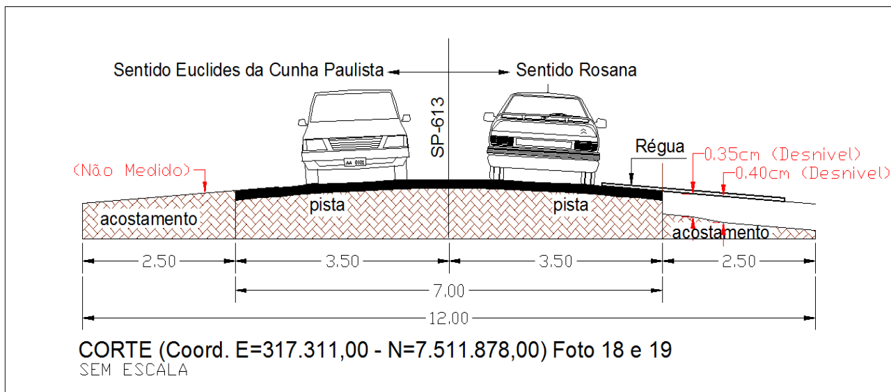
Figura 11 – Desenho do Corte da Rodovia Arlindo Bértio (SP-613), demonstrando o desnível da Rodovia com o seu acostamento do lado direito no sentido Euclides da Cunha Paulista à Rosana.
