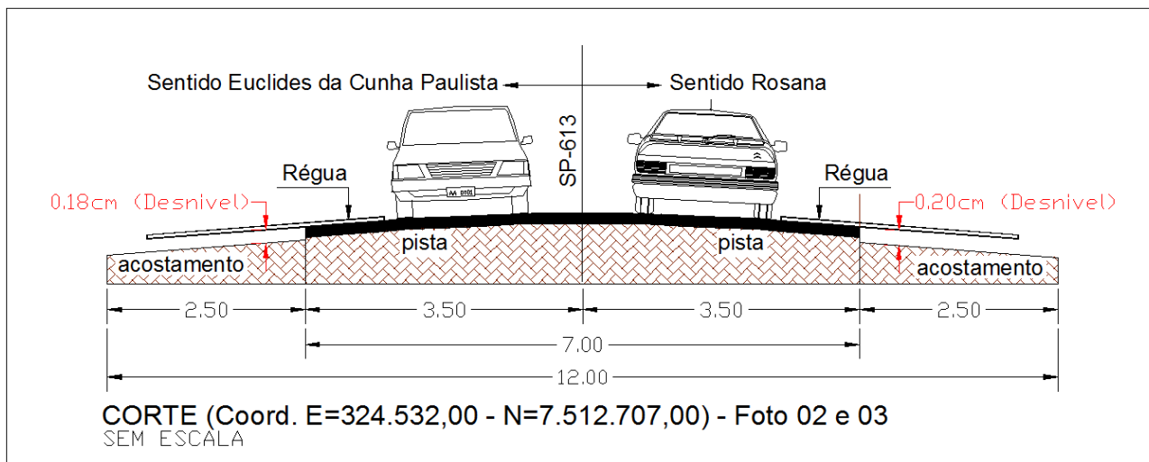
Figura 03 – Desenho do Corte da Rodovia Arlindo Bértio (SP-613), demonstrando o desnível da Rodovia com o seu acostamento do lado direito e esquerdo no sentido Euclides da Cunha Paulista à Rosana.
