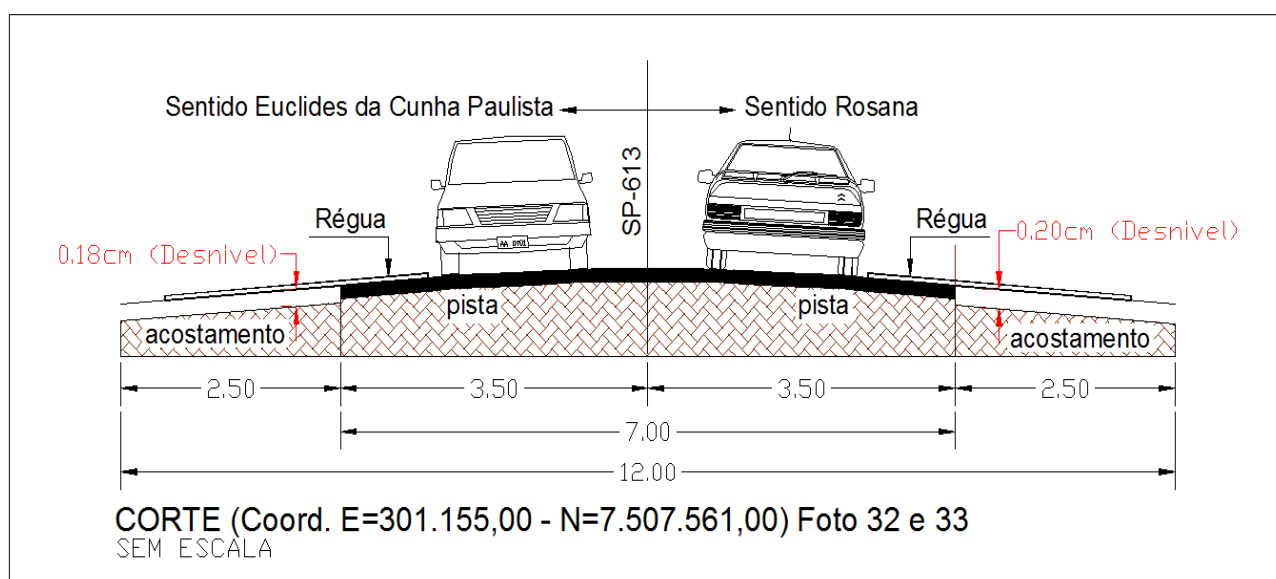
Figura 20 – Desenho do Corte da Rodovia Arlindo Bértio (SP-613), demonstrando o desnível da Rodovia com o seu acostamento do lado direito e esquerdo no sentido Euclides da Cunha Paulista à Rosana.
